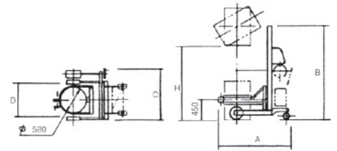
▲ 유압전동식 HDL-3E
